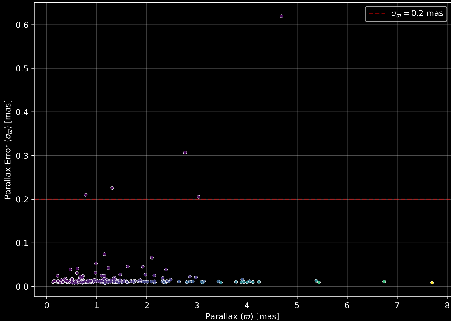
GALAH DR4 Field: [3405] Parallax Quality (n= 253)
