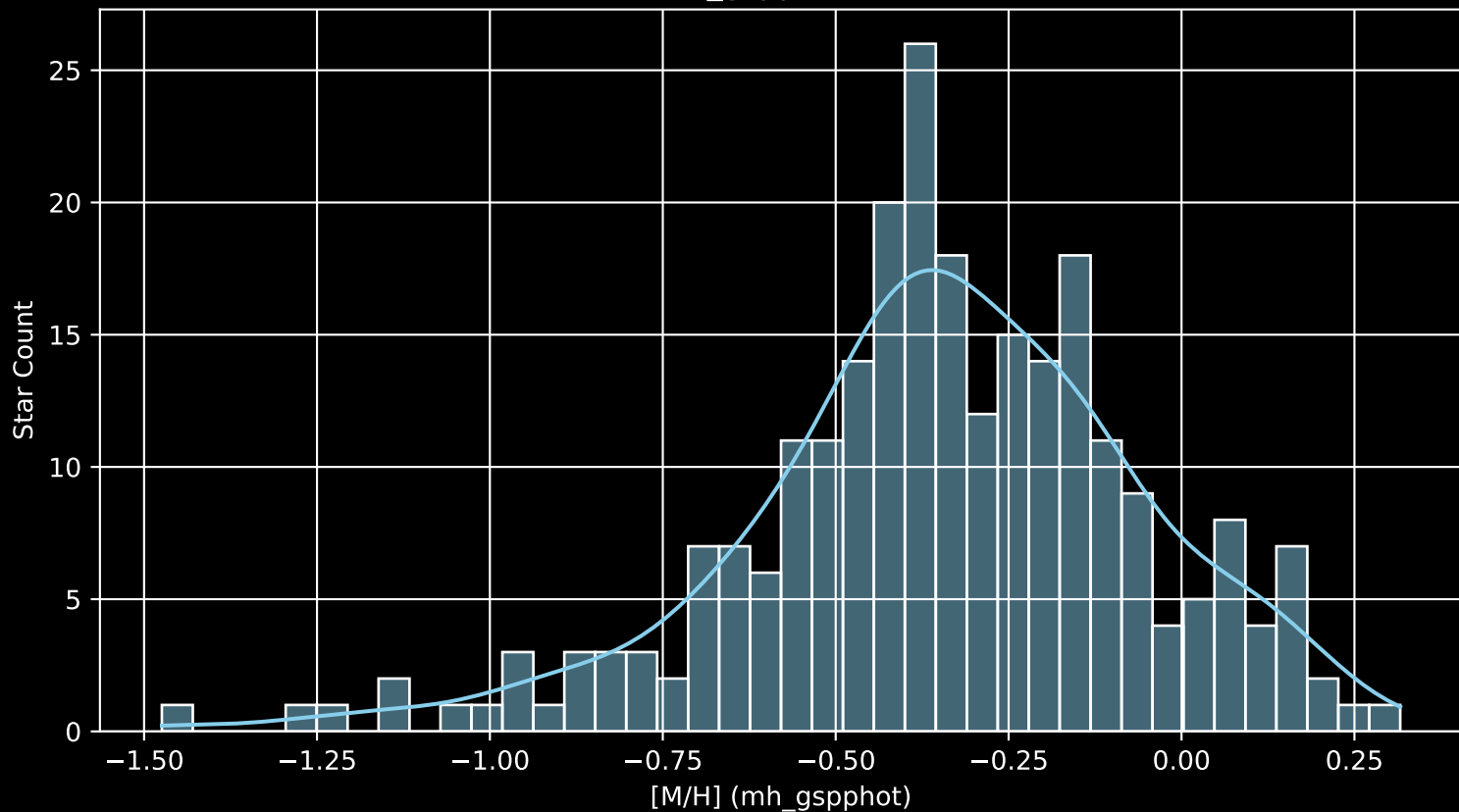
GALAH DR4 Field: [3405] [M/H] (mh_gspphot) (n= 253)
