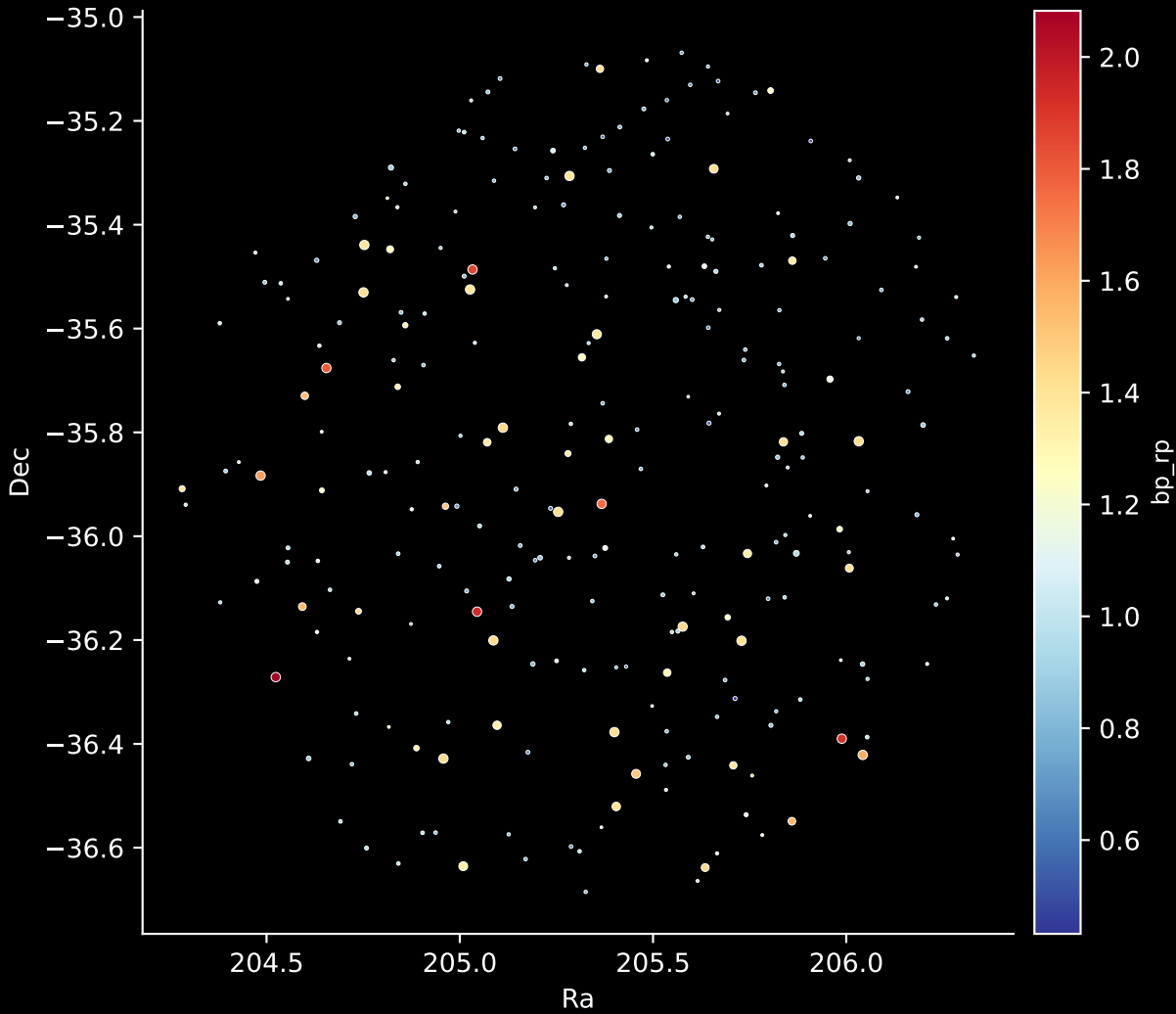
GALAH DR4 Field: [3405] Stars: 253
