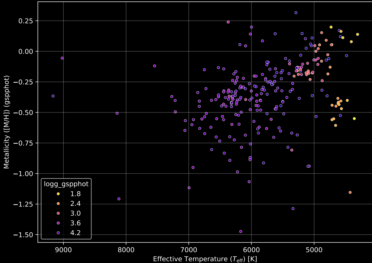
GALAH DR4 Field: [3405] Stellar Population Parameters (n= 253)
