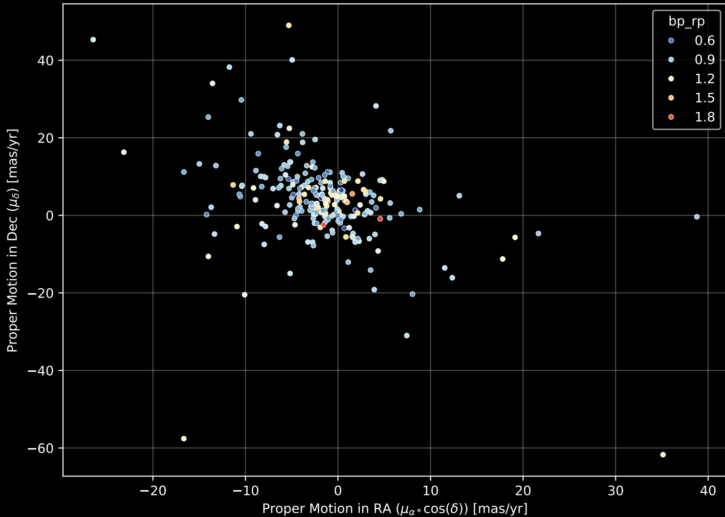
GALAH DR4 Field: [3405] Proper Motion Diagram (n= 253)
